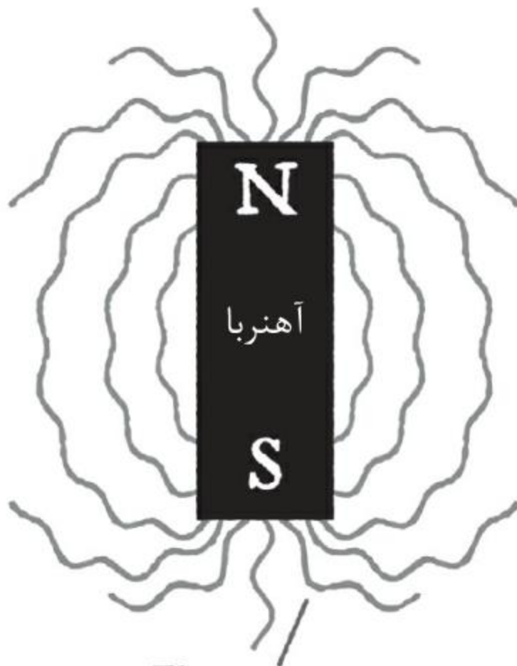
میدان الکترومغناطیسی
