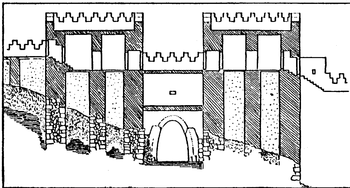
شکل ۵۴: بخش طولی از دروازه غربی سفلا در ختّه، بنابر نظر پوخشتاین. این طرح که متکی بر بازسازی حدسی است، ساختمان عظیم دروازه و همچنین روشی را نشان می‌دهد که دروازه و دیوار را در زمین سربالا می‌ساختند.
