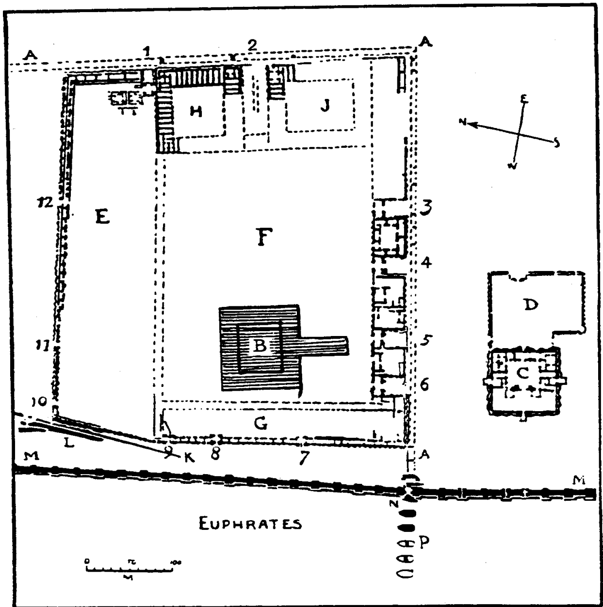
شکل ۲۷: نقشه اِستمن-انکی و اِسگله بنا برگفته و تزل. A: راه مقدس یا کوچه رژه. B: اِستمن-انکی زیگورات با برج معبد بابل. C: اِسگله، معبد مردوک. D: ضمیمه شرقی برای اِسگله. E: حیاط شمالی محوطه‌های مقدس. F: حیاط عمده G: حیاط غربی. H، J: مخازن معبد. K: دیوار آراختو. L: دیوار نبوکدنصر. M: دیوار نبونید در کنار رود. N: دروازه در دیوار کنار رود. P: پایه‌های سنگی پل بر روی فرات. ۱-۱۲: مداخله‌ایی برای پریلوسها محوطه مقدس. شماره ۲، موقعیت مدخل اصلی را نشان می‌دهد.
