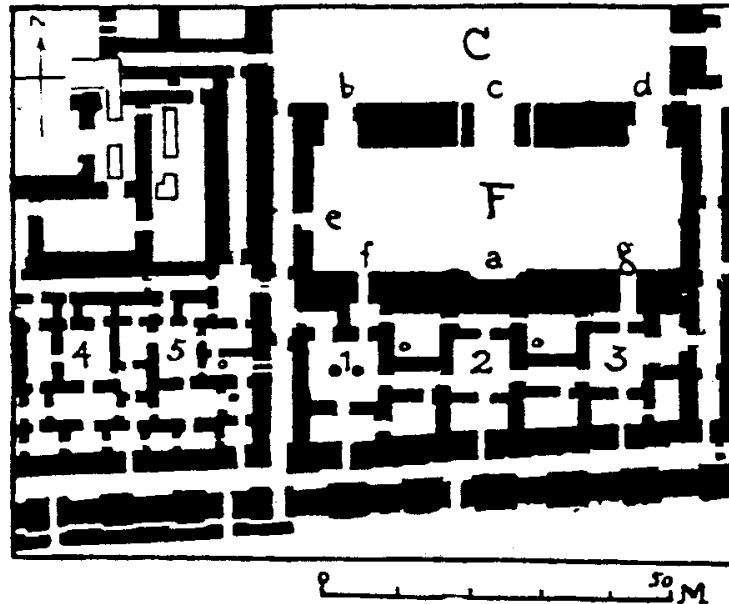
شکل ۹: نقشه اتاق تاجگذاری نبوکدنصر دوم و بخشی از قصر خصوصی. پتابه گفته کول بدوی. C: حیاط بزرگ. F: اتاق تاجگذاری. a: تورفتگی در دیوار اتاق تاجگذاری. d-sb: مدخلهای اتاق تاجگذاری از طرف حیاط. g-e: مدخلها از کنار و پشت. ۱-۳: حیاطهای باز، که در پیرامون آنها اتاقهایی برای خدمت به پادشاه ساخته شده بود. ۴، ۵: دیوارهای باز در زاویه جنوب شرقی قصر خصوصی.
