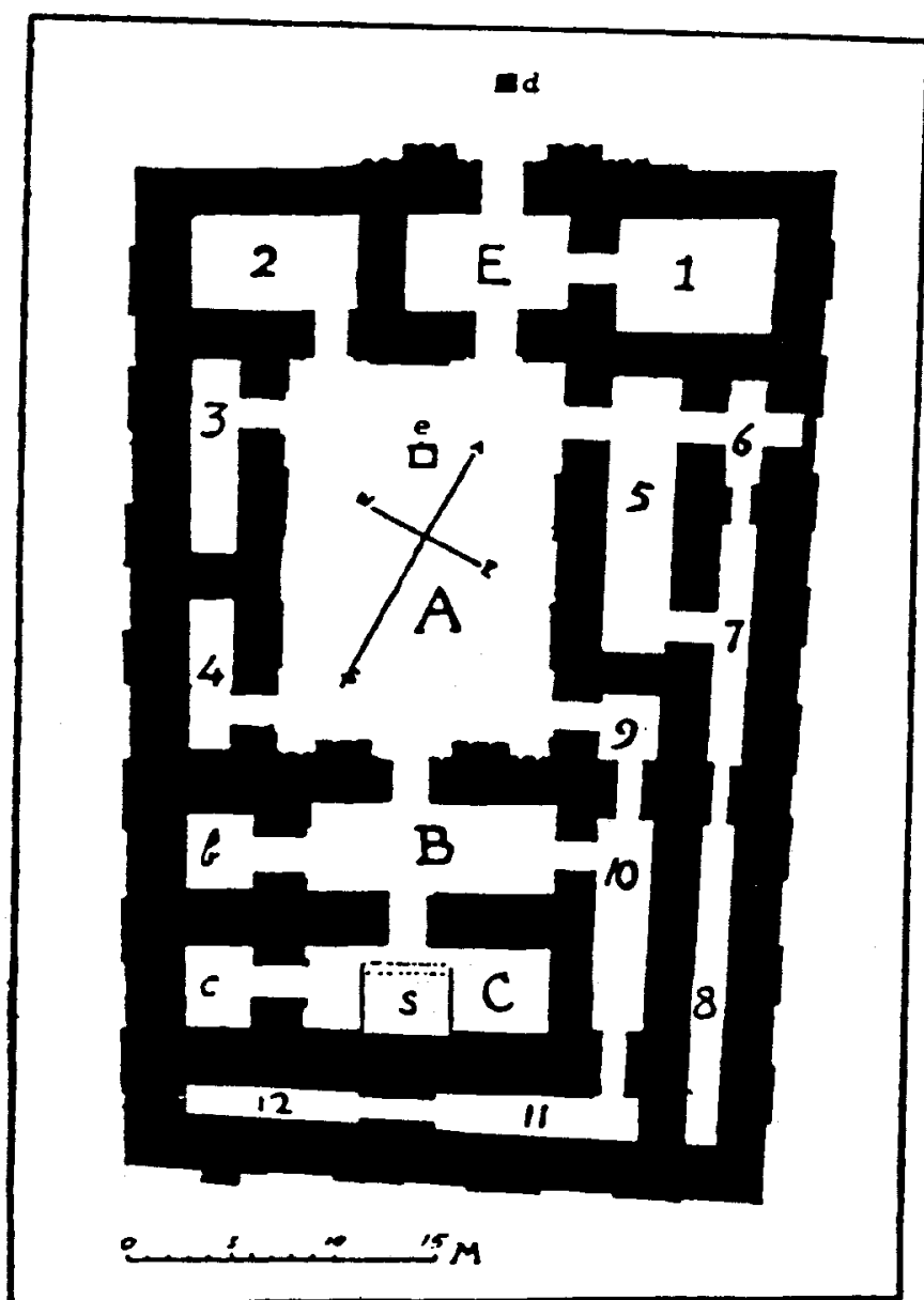
شکل ۲۰: طرح ا- معبد، معبد الالهه نین-معبد بنابر گفته آندریاس. A: حیاط باز. B: اتاق کفش‌کن جلو ضریح. C: ضریح. E: اتاق ورودی یا دالان منتهی به معبد. b: اتاق عبادت برای اتاق کفش‌کن. C: اتاقی برای ضریح. d: محراب خشتی. e: چاه. S: شاه‌نشین برای تندیس نین-معبد. ۱: اتاق باربران. ۲-۴: اتاقهای کاهنان یا مخازن. ۵، ۶، ۹، ۱۰: اتاقهای منتهی به راهروهای باریک. ۷، ۸، ۱۱، ۱۲: راهروهای باریک احتمالاً دارای پله یا نرده برای رفتن به بام.
